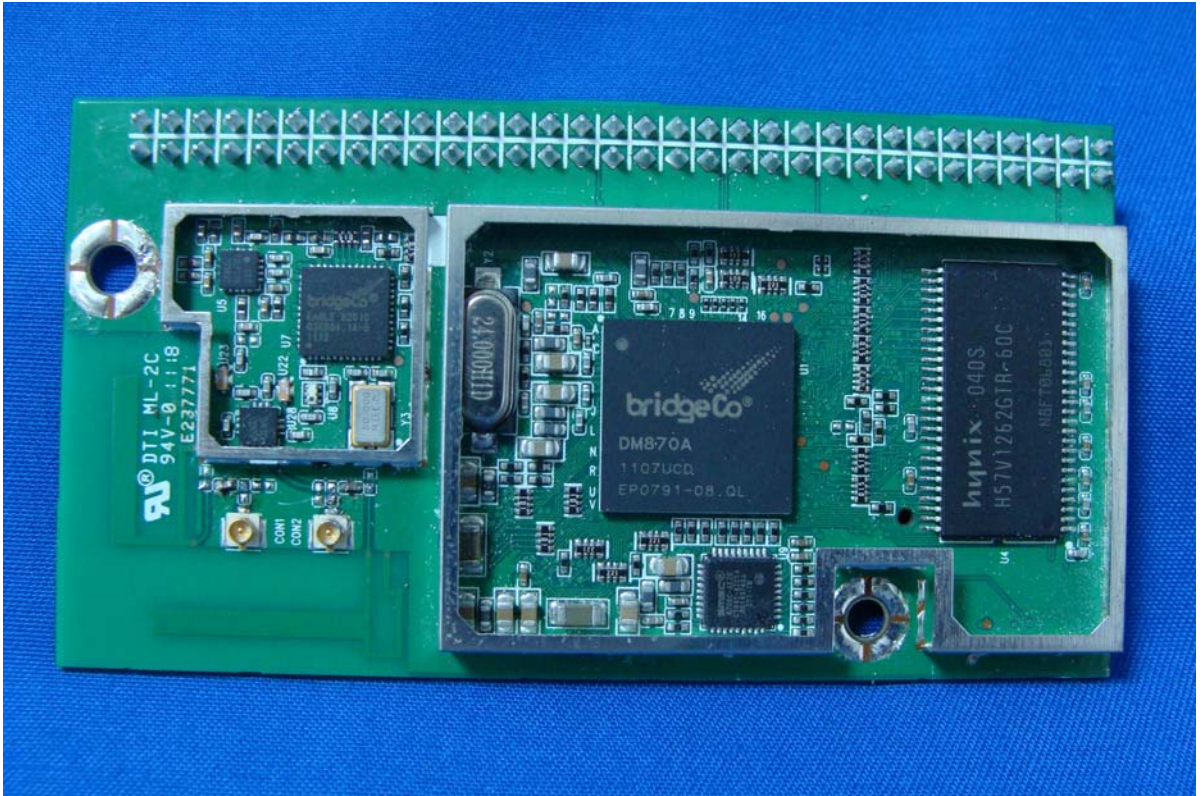
(6) EUT Photo
