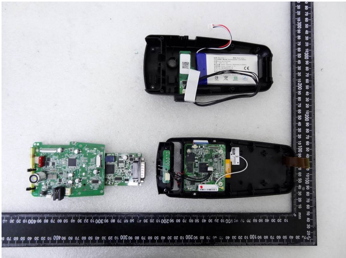
EUT-2.
