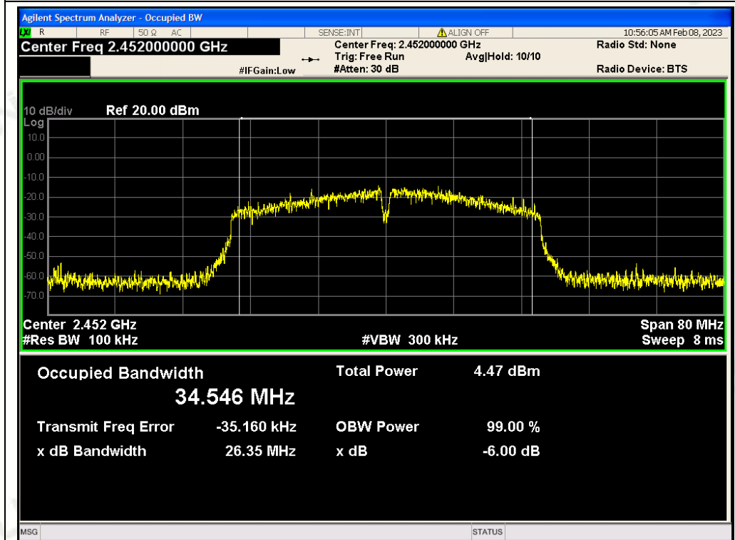
CH09: 2452MHz
