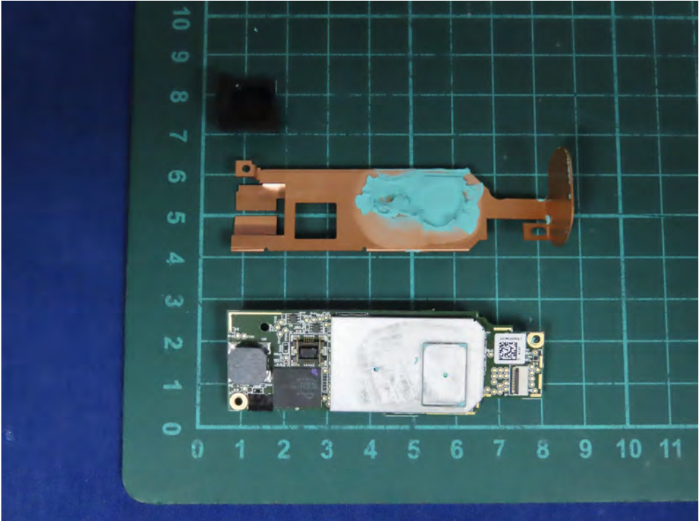
(20) EUT Photo
