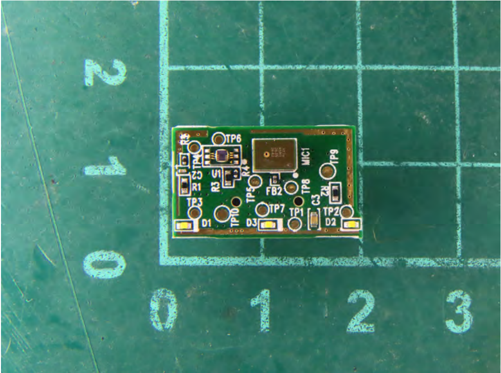
(16) EUT Photo
