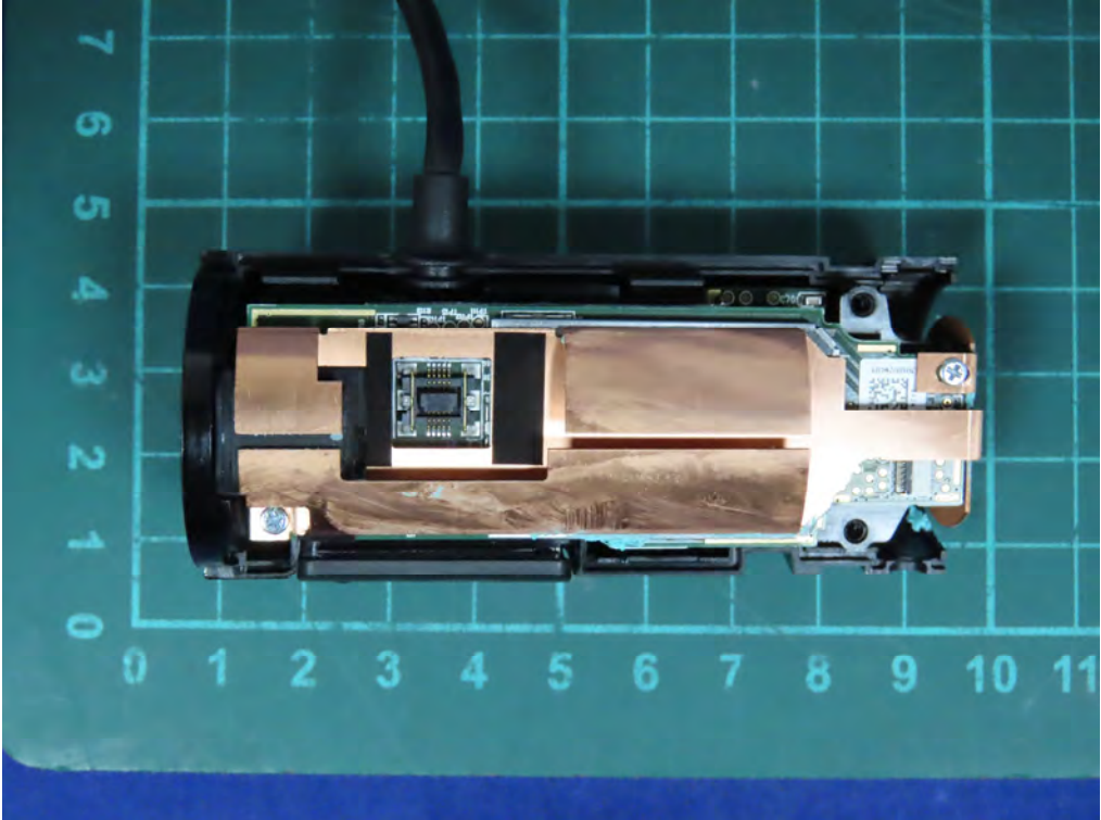
(17) EUT Photo
