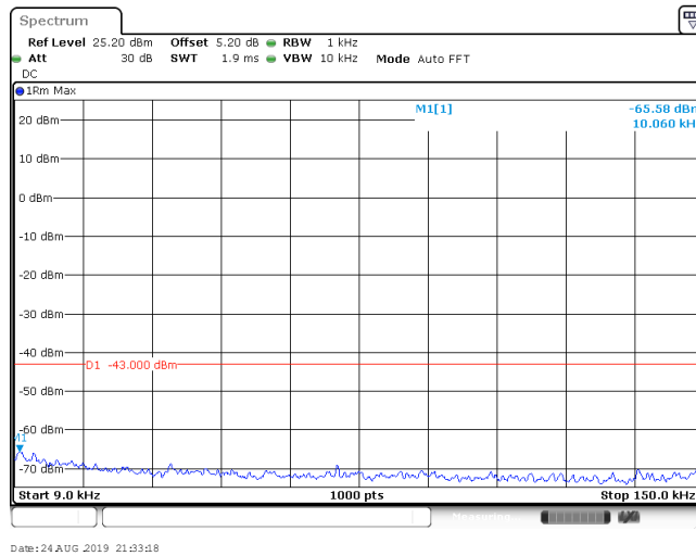
Band IV_1312
