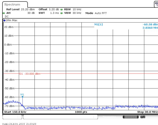
Band IV_1312
