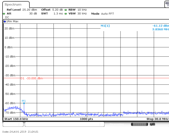
Band IV_1312
