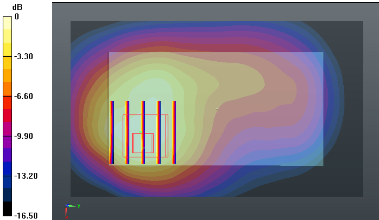
0 dB = 1.400\text{mW/g}
