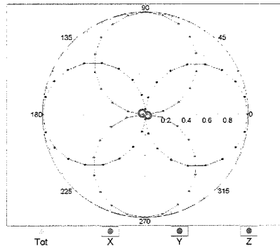
f=2500 MHz,R22,0°
