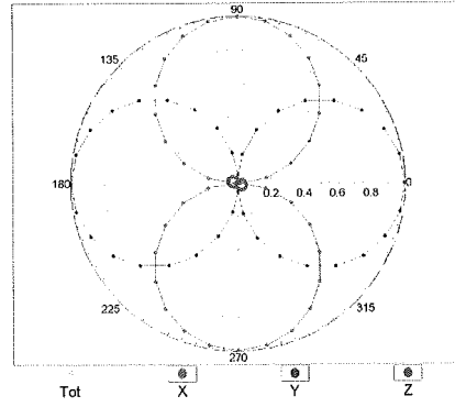
f=2500 MHz,R22,0°
