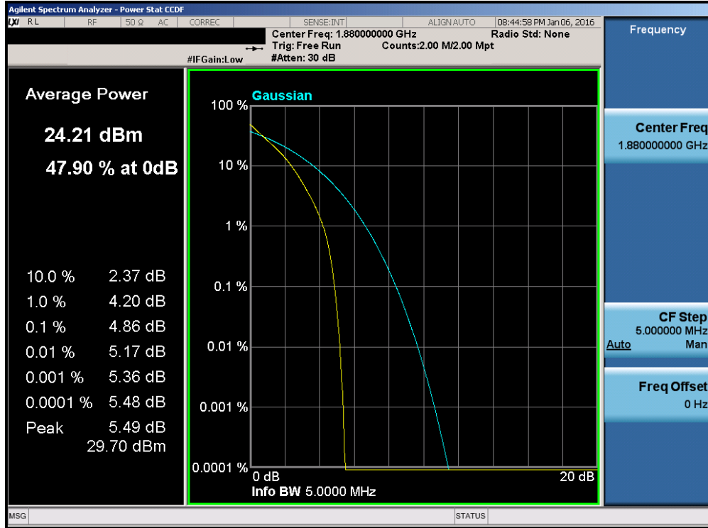
Plot 7-203. PAR Plot (Band 2 – 5.0MHz QPSK – RB Size 25)
