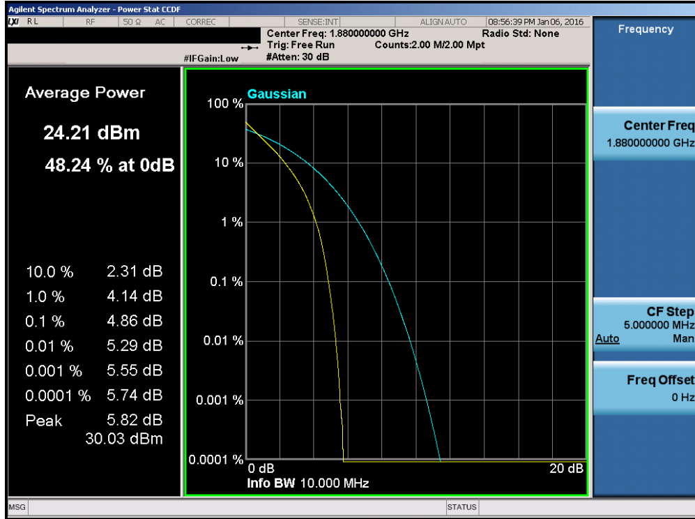
Plot 7-205. PAR Plot (Band 2 – 10.0MHz QPSK – RB Size 50)
