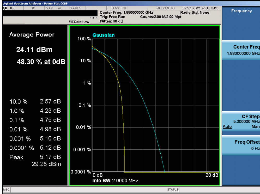
Plot 7-199. PAR Plot (Band 2 – 1.4MHz QPSK – RB Size 6)
