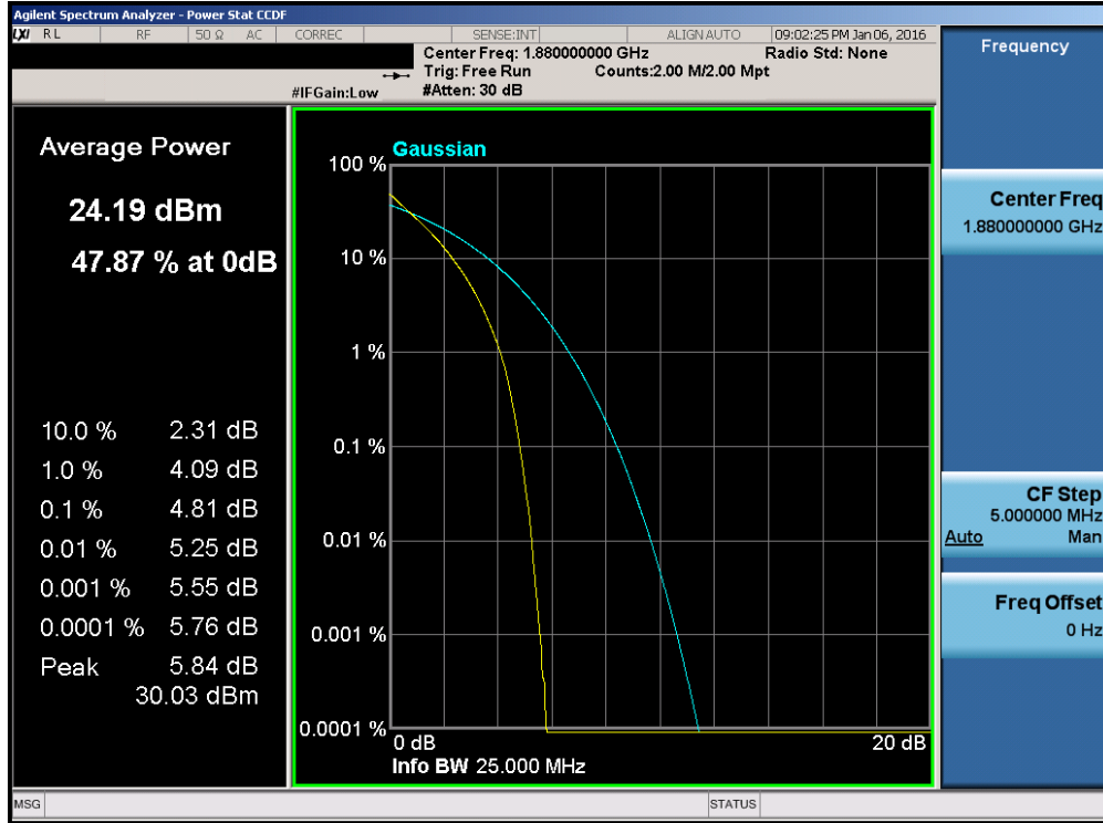
Plot 7-209. PAR Plot (Band 2 – 20.0MHz QPSK – RB Size 100)
