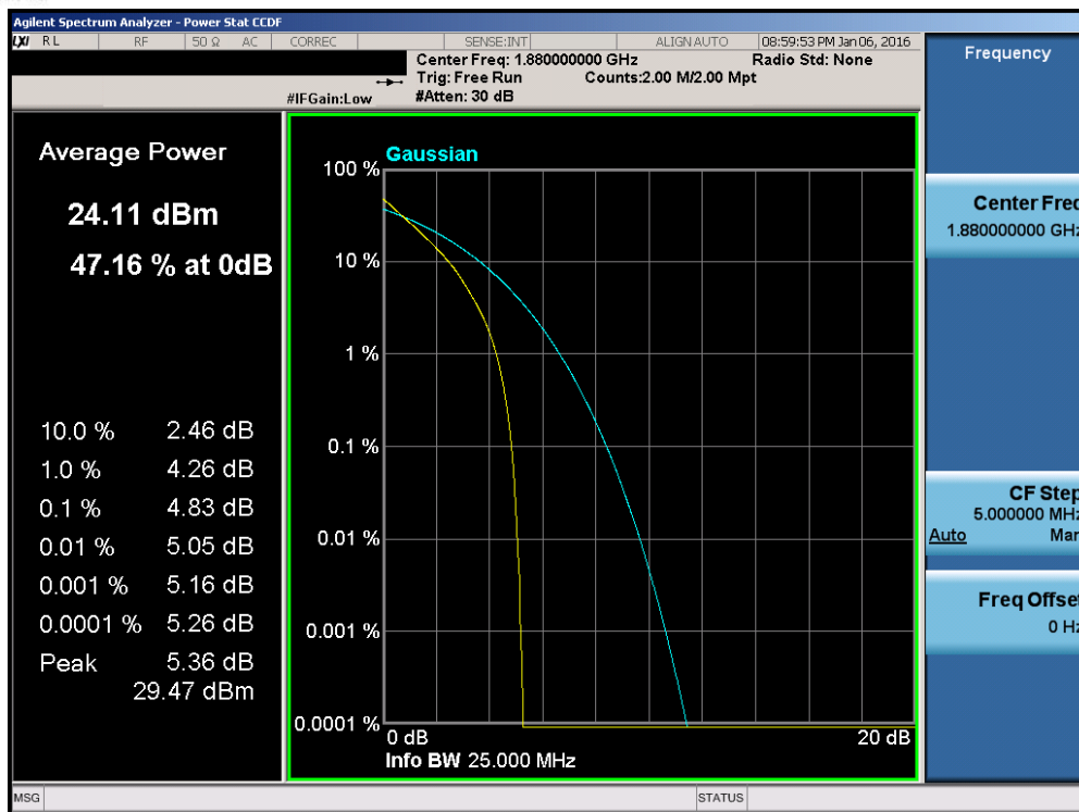
Plot 7-207. PAR Plot (Band 2 – 15.0MHz QPSK – RB Size 75)
