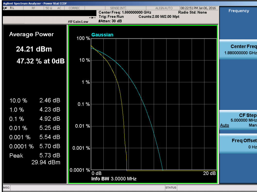
Plot 7-201. PAR Plot (Band 2 – 3.0MHz QPSK – RB Size 15)
