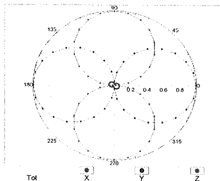
f=2500 MHz,R22,0°
