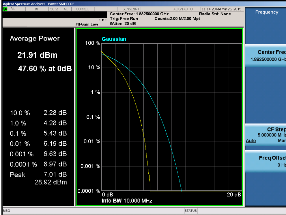
Plot 6-178. PAR Plot (Band 25 – 10.0MHz QPSK – RB Size 50)
