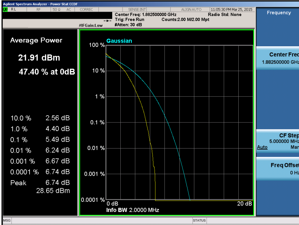
Plot 6-172. PAR Plot (Band 25 – 1.4MHz QPSK – RB Size 6)
