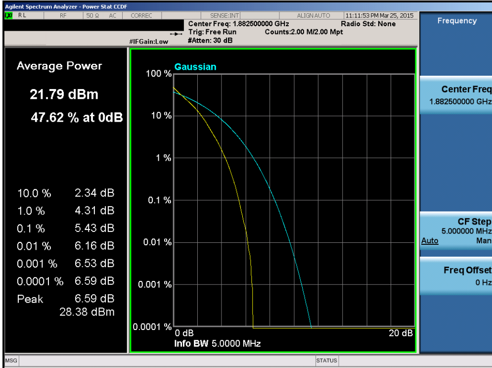
Plot 6-176. PAR Plot (Band 25 – 5.0MHz QPSK – RB Size 25)
