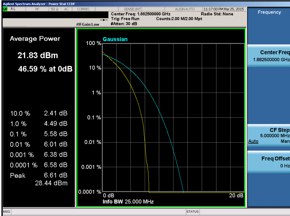
Plot 6-180. PAR Plot (Band 25 – 15.0MHz QPSK – RB Size 75)
