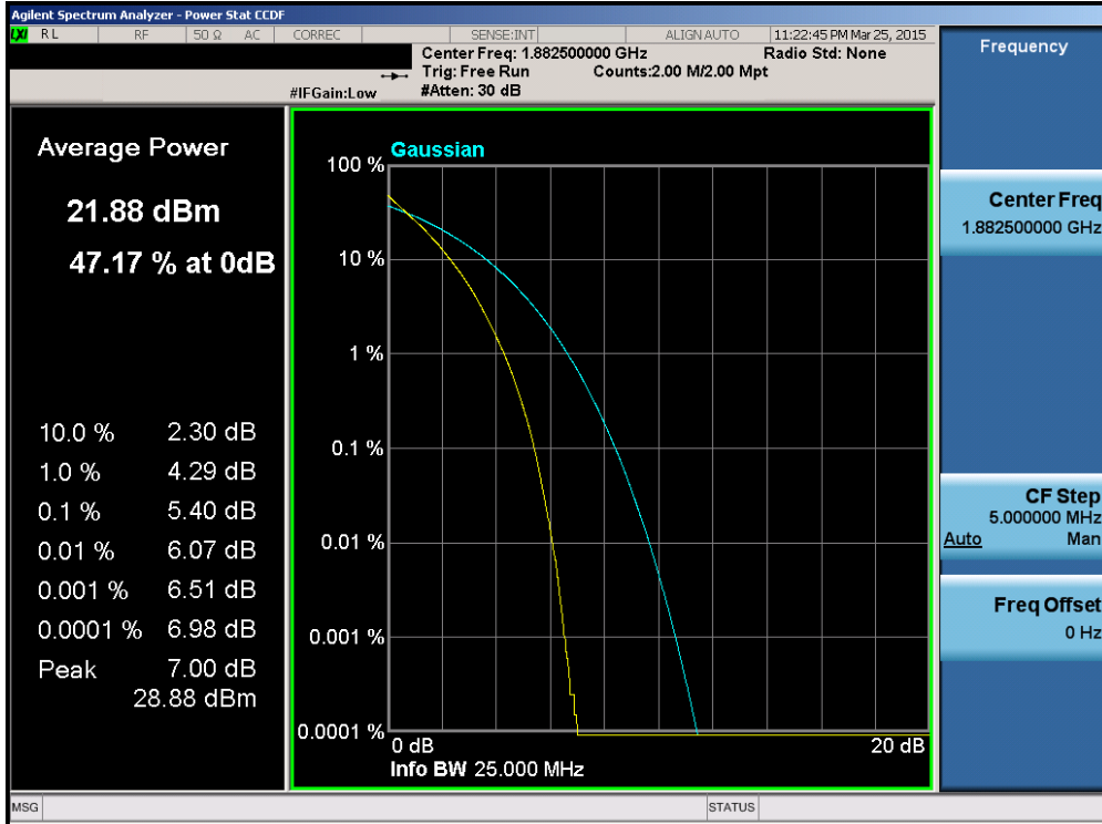
Plot 6-182. PAR Plot (Band 25 – 20.0MHz QPSK – RB Size 100)
