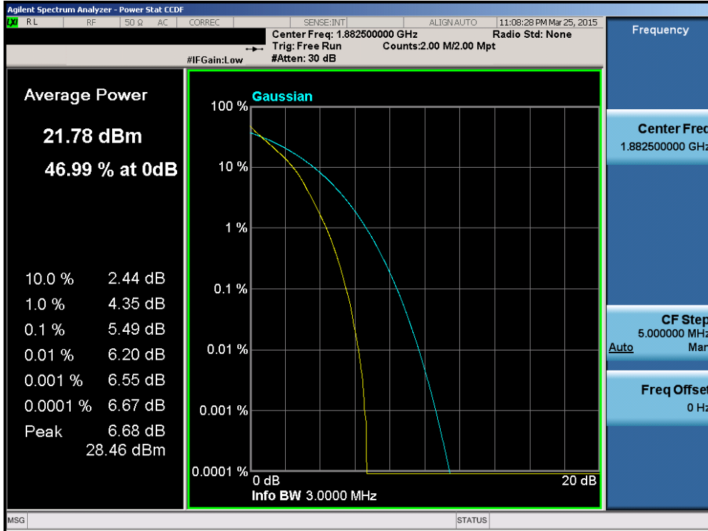
Plot 6-174. PAR Plot (Band 25 – 3.0MHz QPSK – RB Size 15)
