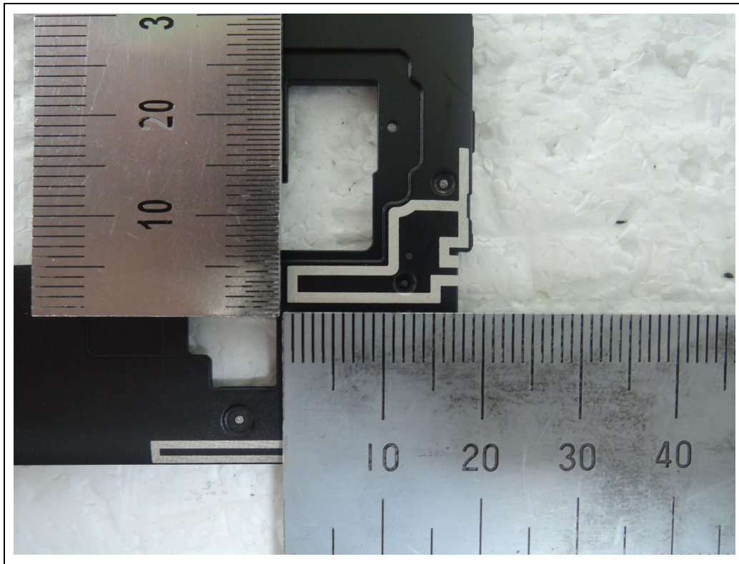
<Antenna>
