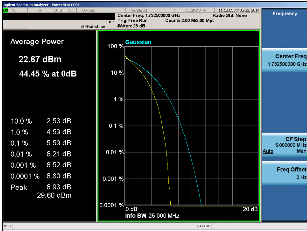
Plot 6-126. PAR Plot (Band 4 – 20.0MHz – QPSK – RB Size 100)
