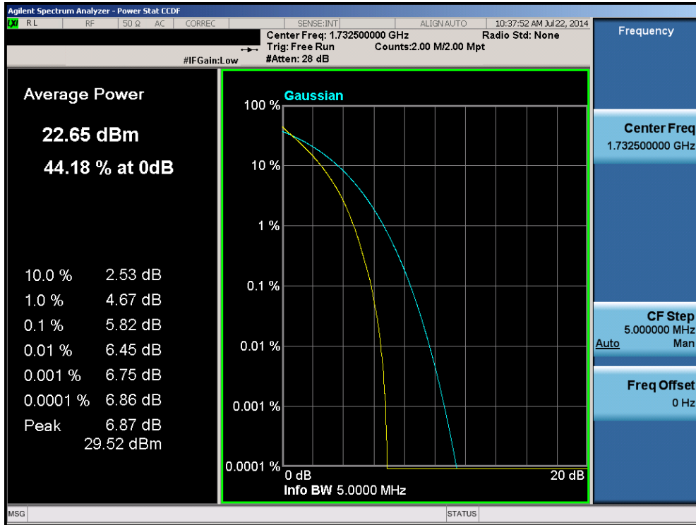
Plot 6-120. PAR Plot (Band 4 – 5.0MHz QPSK – RB Size 25)
