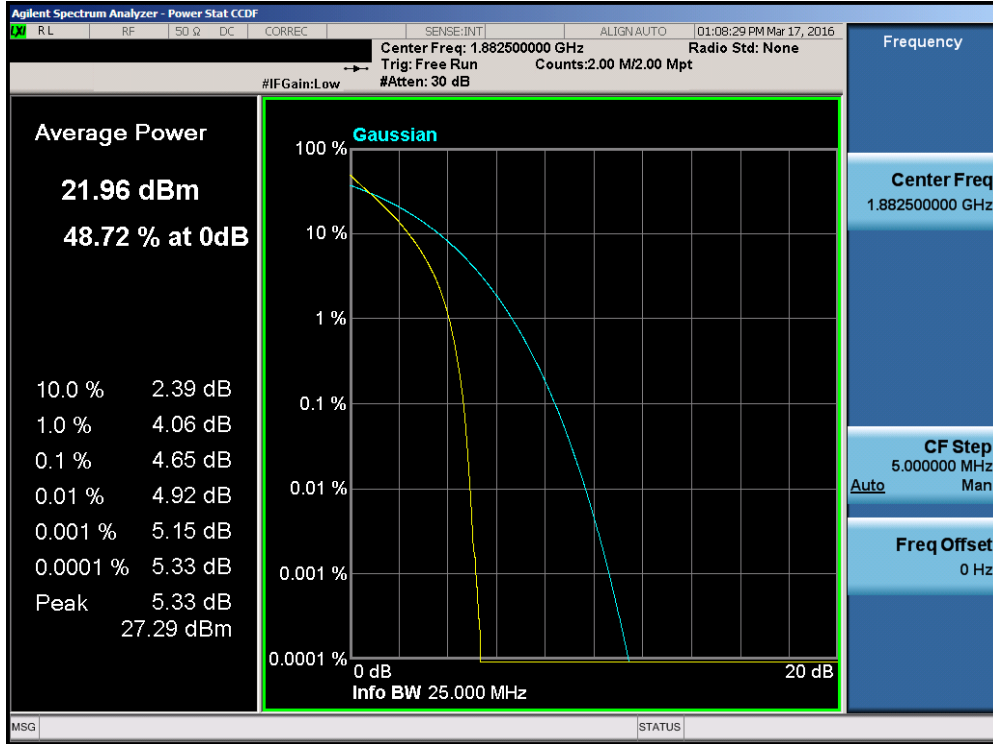
Plot 7-190. PAR Plot (Band 25 – 15.0MHz QPSK – RB Size 75)
