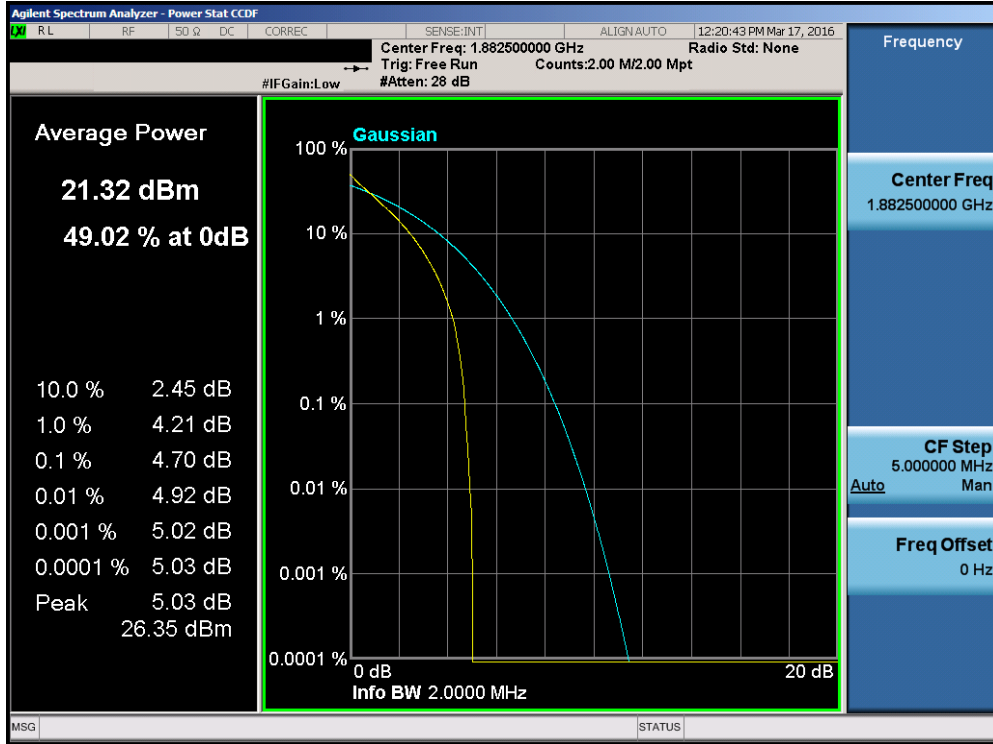
Plot 7-182. PAR Plot (Band 25 – 1.4MHz QPSK – RB Size 6)
