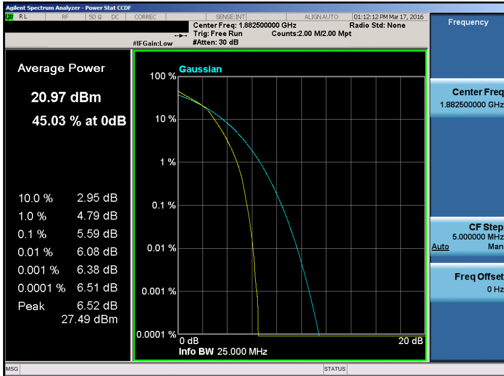
Plot 7-193. PAR Plot (Band 25 – 20.0MHz 16-QAM – RB Size 100)
