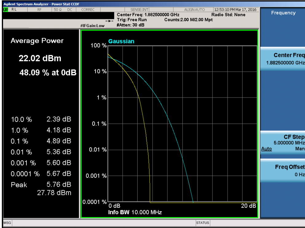
Plot 7-188. PAR Plot (Band 25 – 10.0MHz QPSK – RB Size 50)
