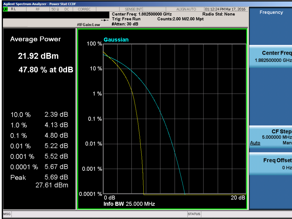
Plot 7-192. PAR Plot (Band 25 – 20.0MHz QPSK – RB Size 100)
