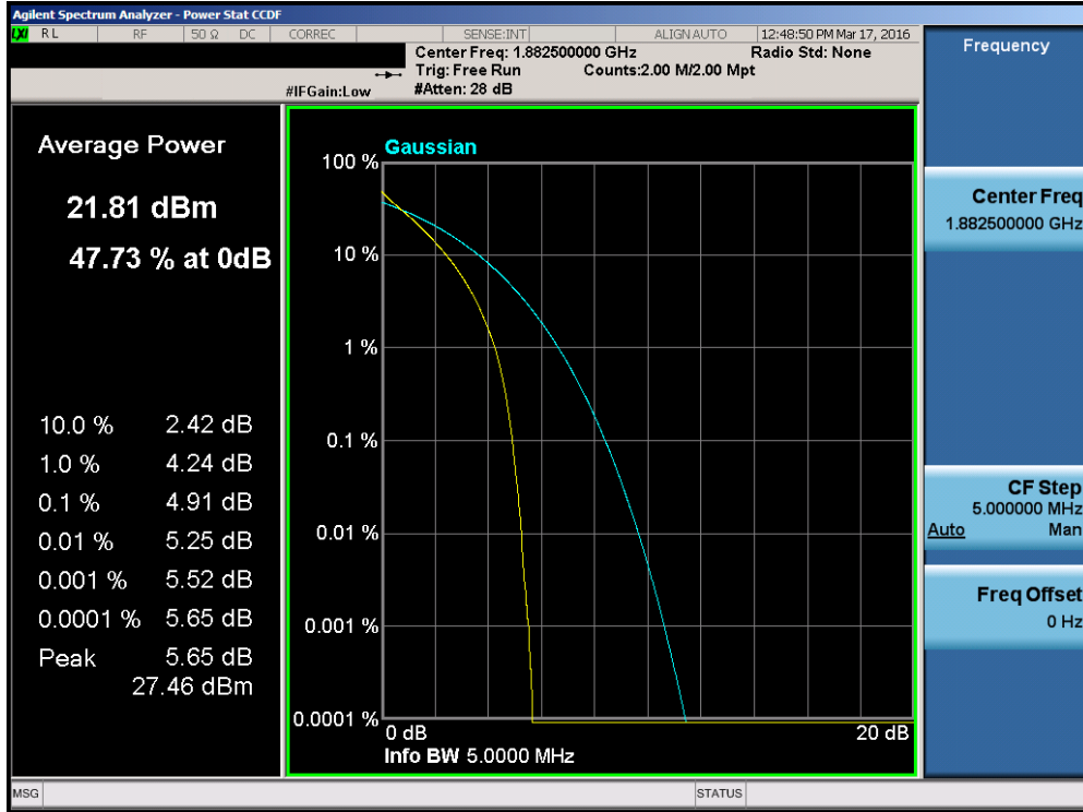
Plot 7-186. PAR Plot (Band 25 – 5.0MHz QPSK – RB Size 25)
