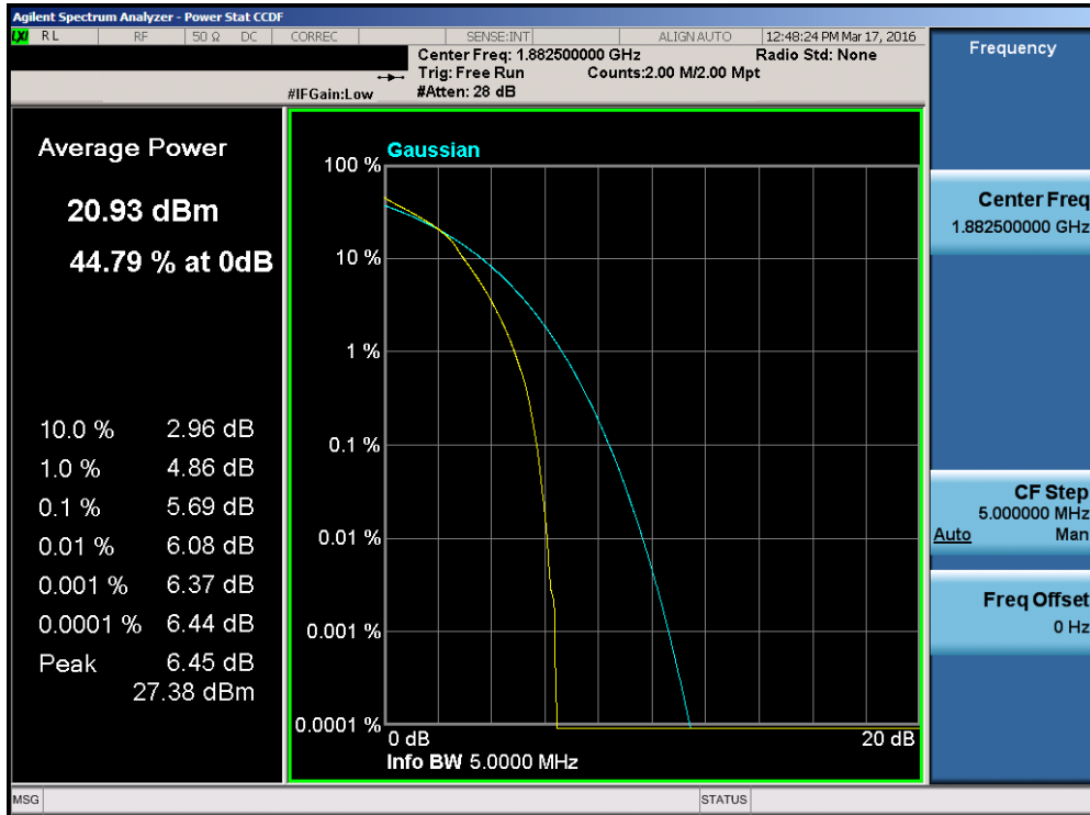
Plot 7-187. PAR Plot (Band 25 – 5.0MHz 16-QAM – RB Size 25)
