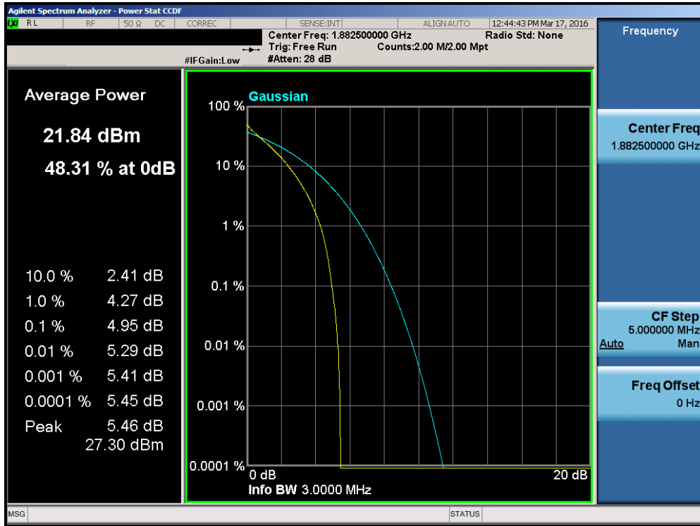
Plot 7-184. PAR Plot (Band 25 – 3.0MHz QPSK – RB Size 15)
