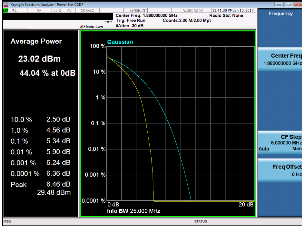
Plot 7-116. PAR Plot (Band 2 – 20.0MHz QPSK – RB Size 100)
