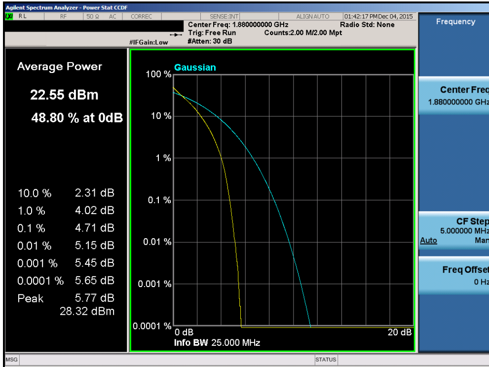
Plot 7-123. PAR Plot (Band 2 – 20.0MHz QPSK – RB Size 100)
