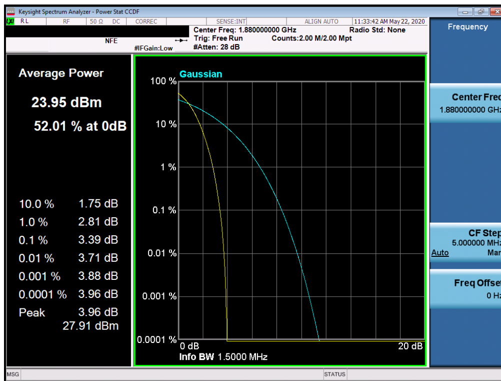
Plot 7-101. PAR Plot (CDMA, Ch. 600)
