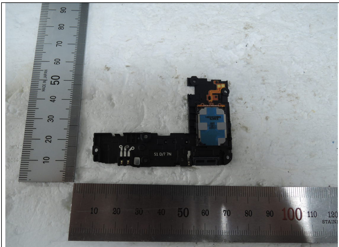
<Antenna>
