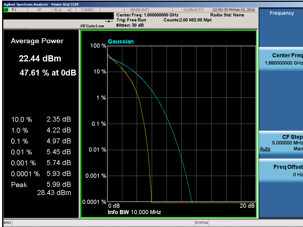
Plot 7-121. PAR Plot (Band 2 – 10.0MHz QPSK – RB Size 50)
