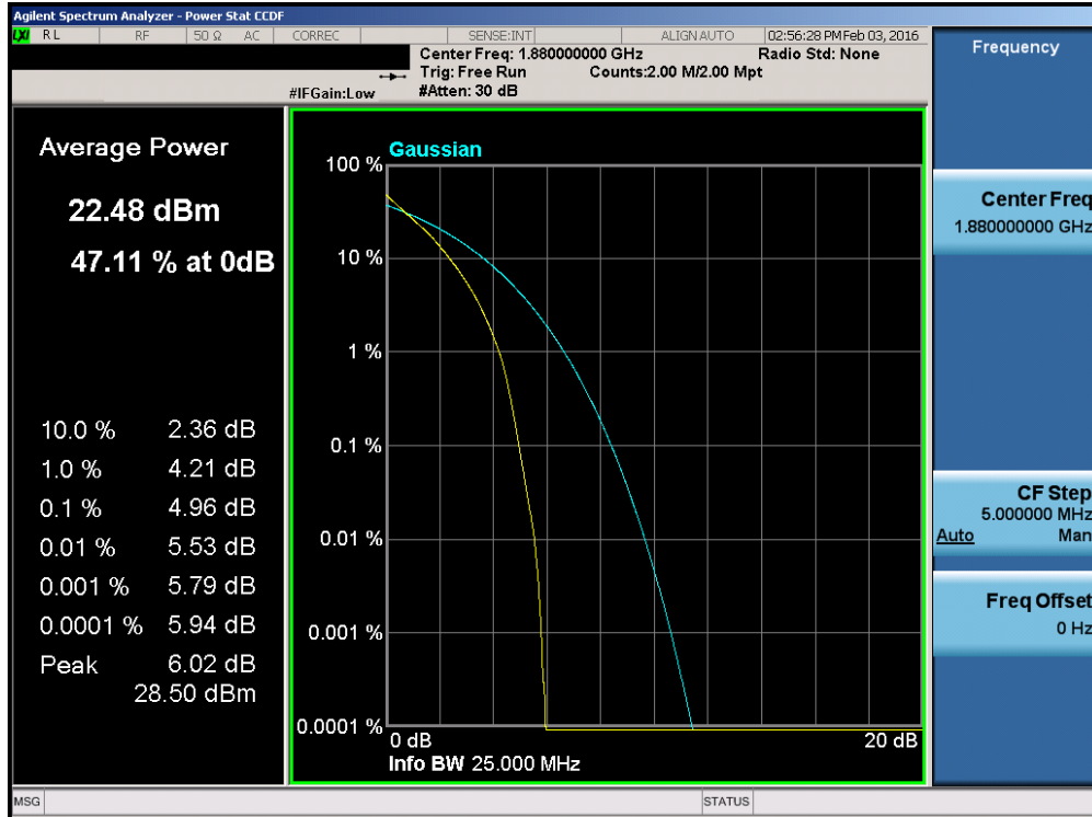
Plot 7-125. PAR Plot (Band 2 – 20.0MHz QPSK – RB Size 100)
