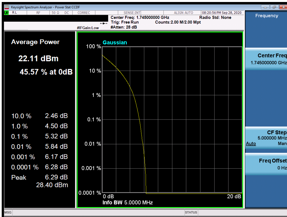
Plot 7-154. PAR Plot (LTE Band 66/4 - 5MHz QPSK - Full RB Configuration)
