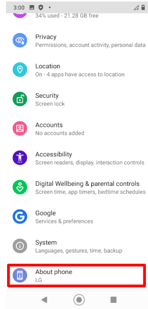
[Step2]
