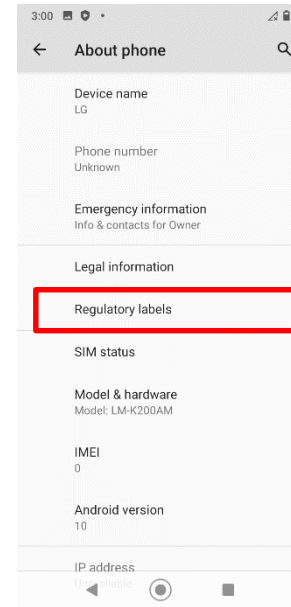
[Step3]
