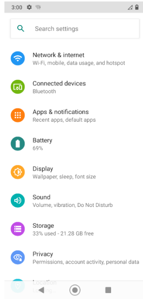
[Step1]
