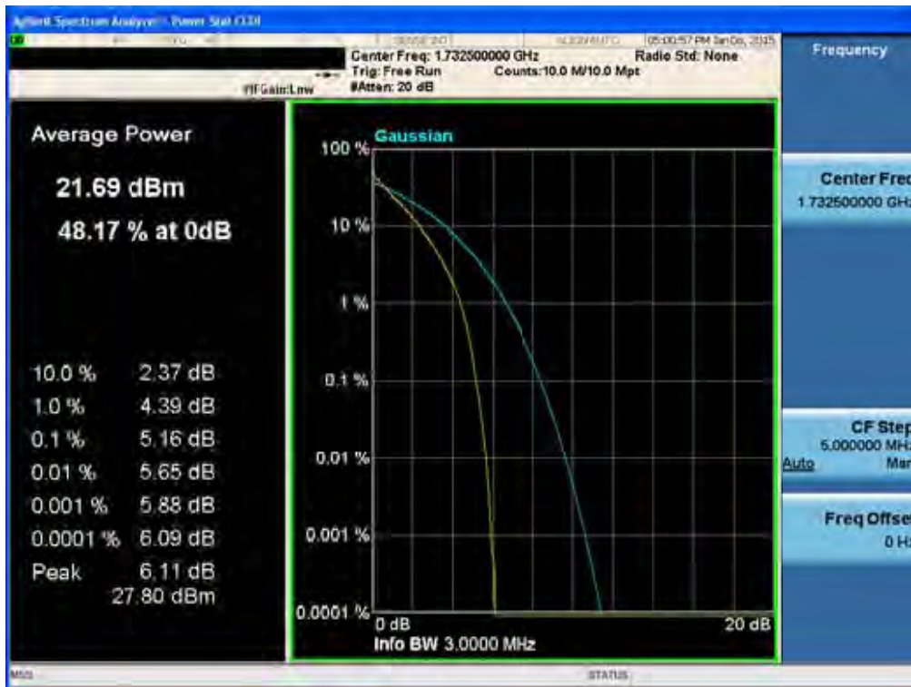
BAND 4. PAR Plot (3M BW_Ch.20175_QPSK_RB15_0)
