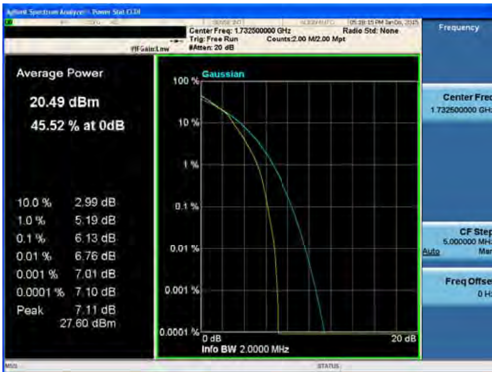
BAND 4. PAR Plot (1.4M BW_Ch.20175_16QAM_RB6_0)
