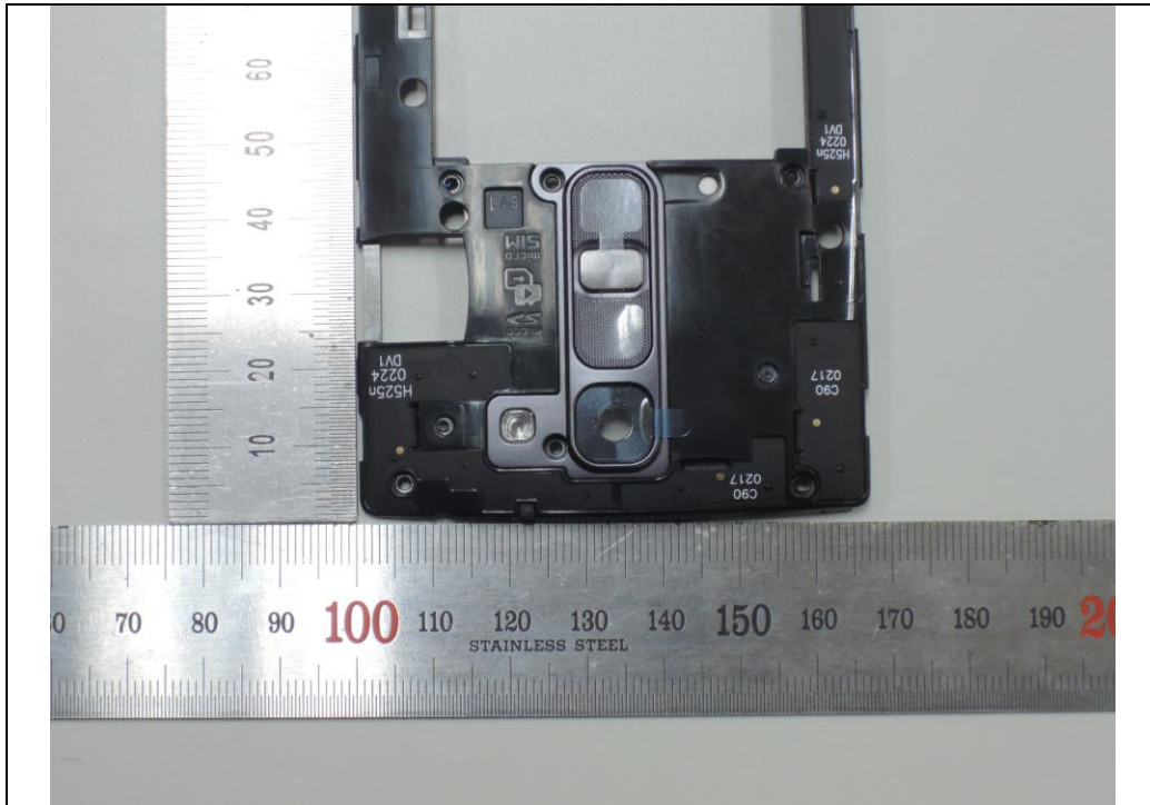
WLAN_BT_GNSS_LTE ANT
