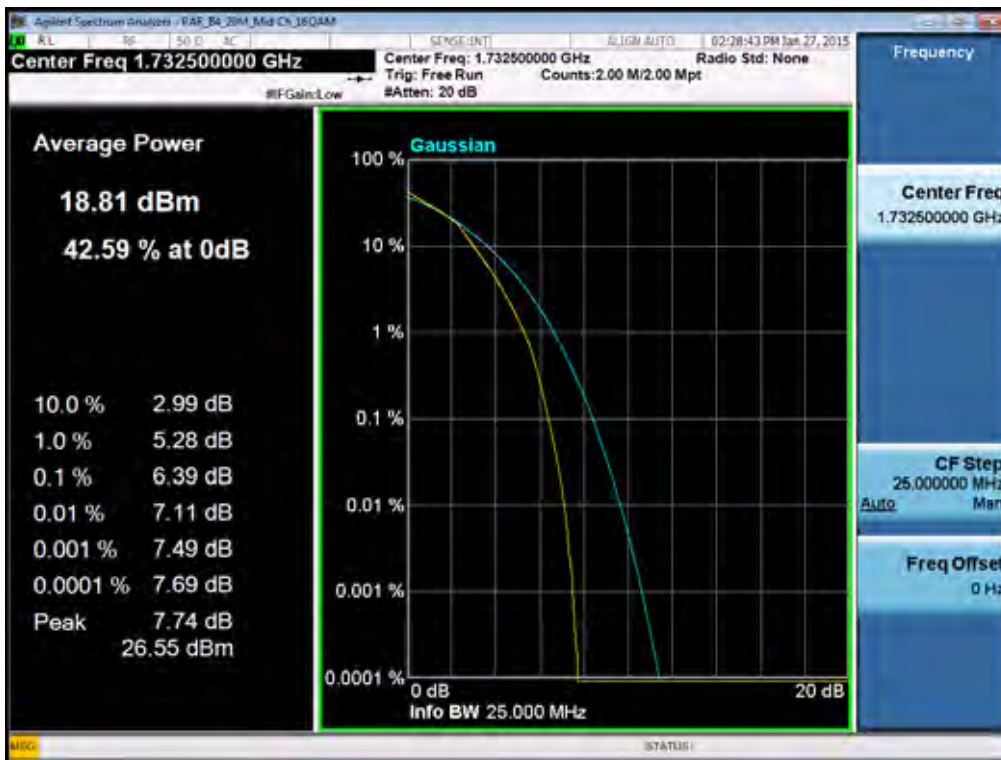
BAND 4. PAR Plot (20M BW_Ch.20175_16QAM_RB100_0)
