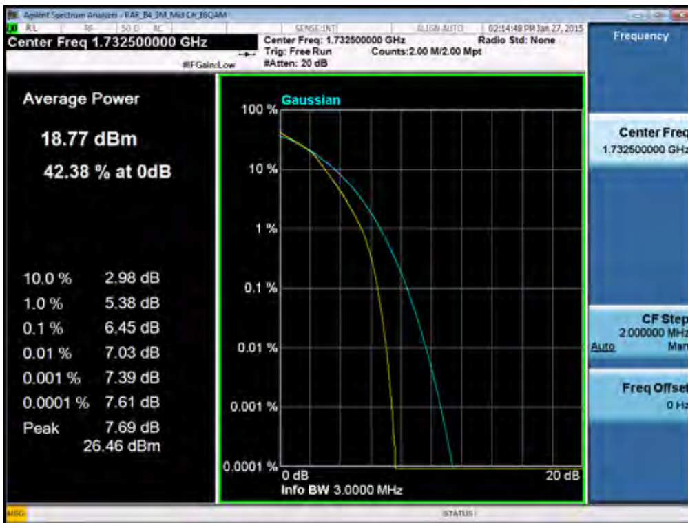
BAND 4. PAR Plot (3M BW_Ch.20175_16QAM_RB15_0)
