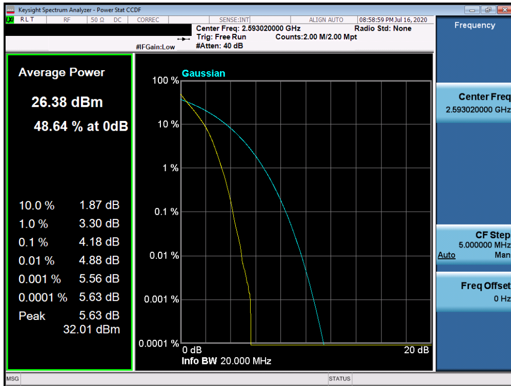
Plot 7-759. PAR Plot (n41 - 20.0MHz DFT-s-OFDM-BPSK - Full RB Configuration)
