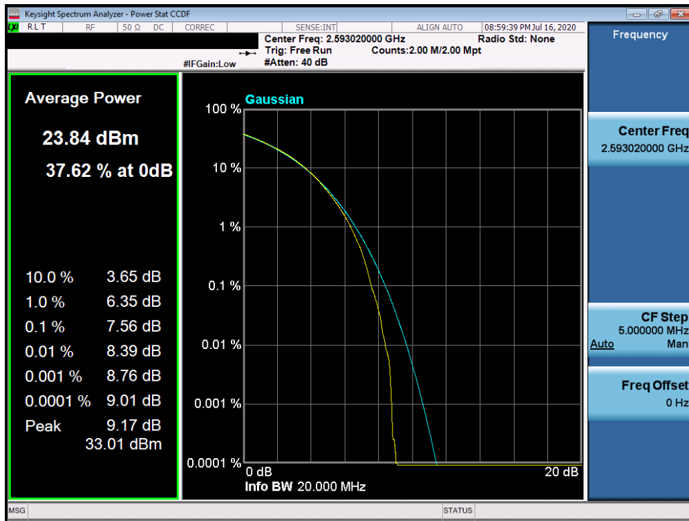
Plot 7-760. PAR Plot (n41 - 20.0MHz CP-OFDM-QPSK - Full RB Configuration)
