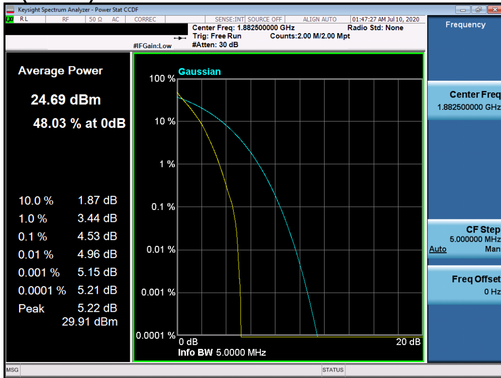
Plot 7-621. PAR Plot (Band n25 - 5.0MHz BPSK - Full RB Configuration)
