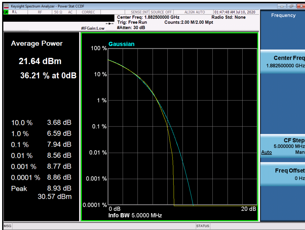
Plot 7-622. PAR Plot (Band n25 - 5.0MHz QPSK - Full RB Configuration)
