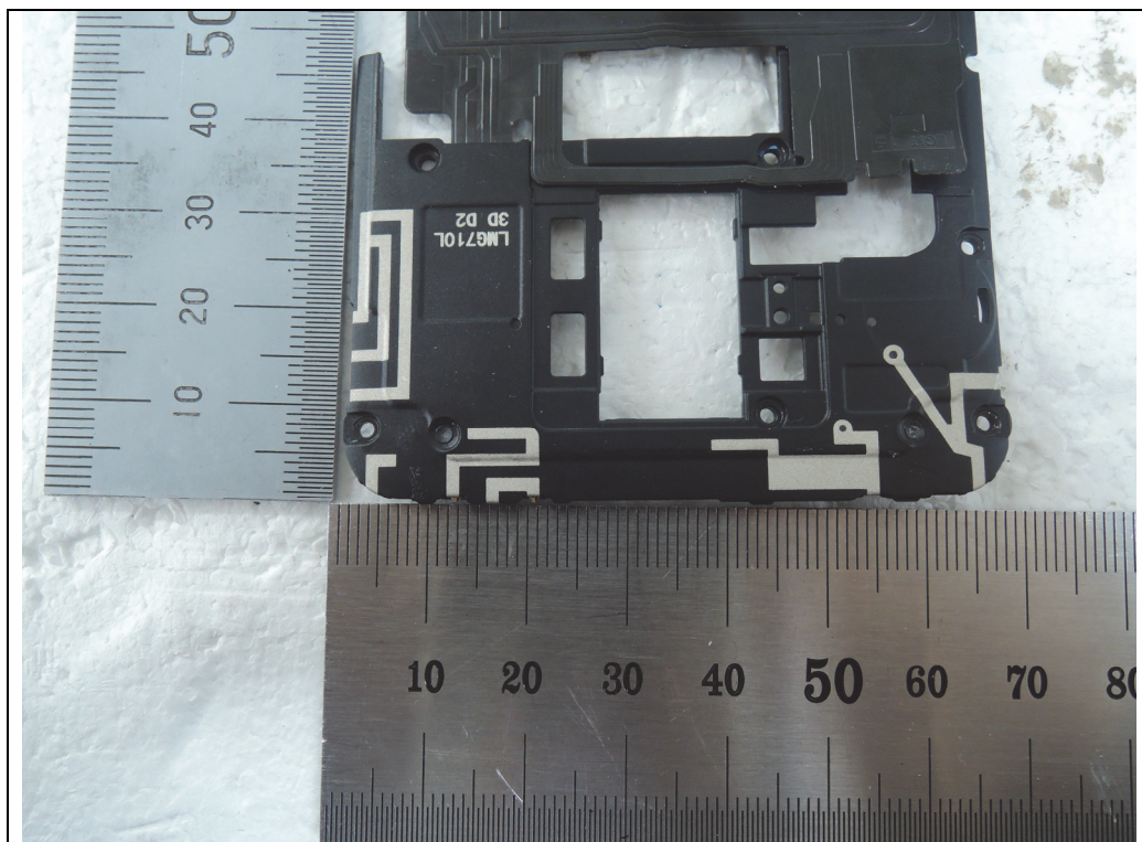
<Antenna 3>
