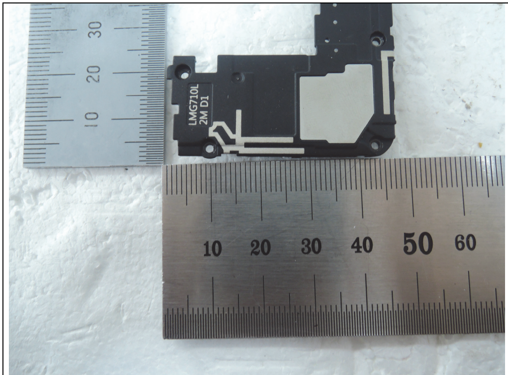
<Antenna 2>
