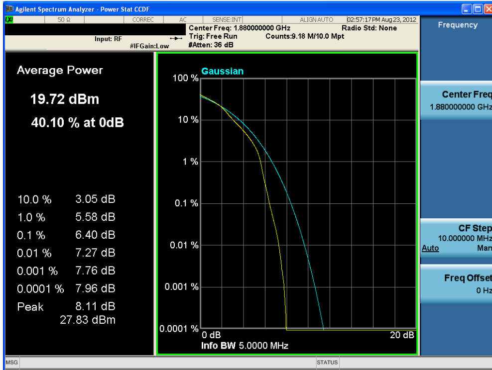
Plot 10-20. PAR Plot (5MHz 16QAM – RB Size 25)
