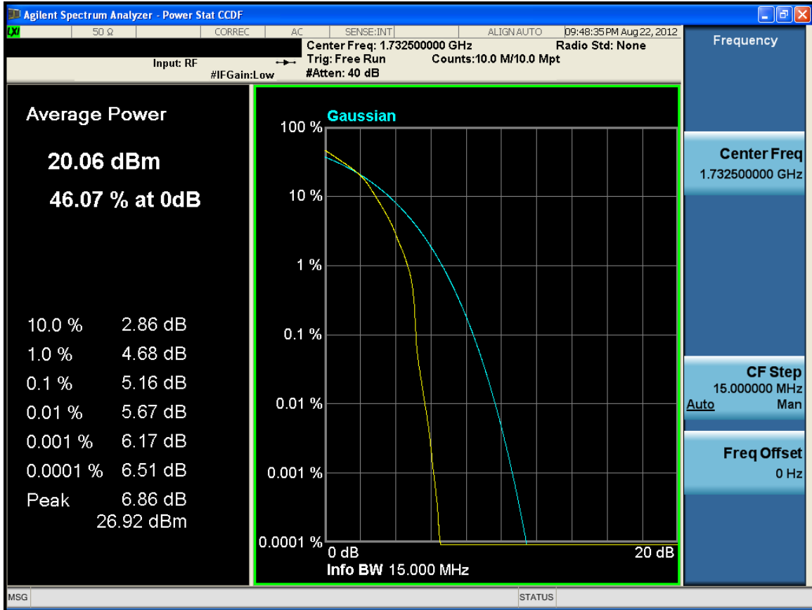
Plot 9-30. PAR Plot (15MHz 16QAM – RB Size 75)
