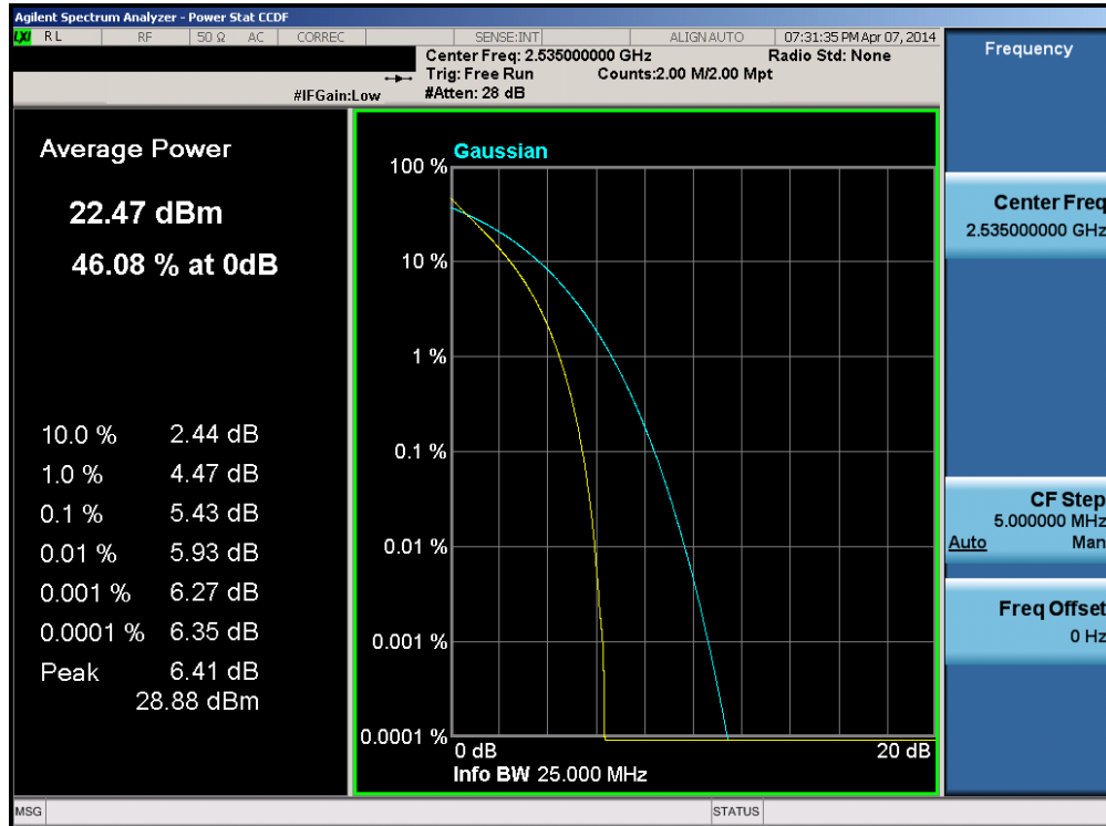
Plot 6-151. PAR Plot (Band 7 – 15.0MHz QPSK – RB Size 75)
