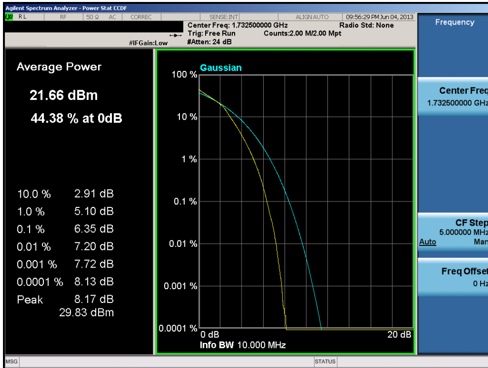
Plot 8-20. PAR Plot (10.0MHz 16-QAM – RB Size 50)
