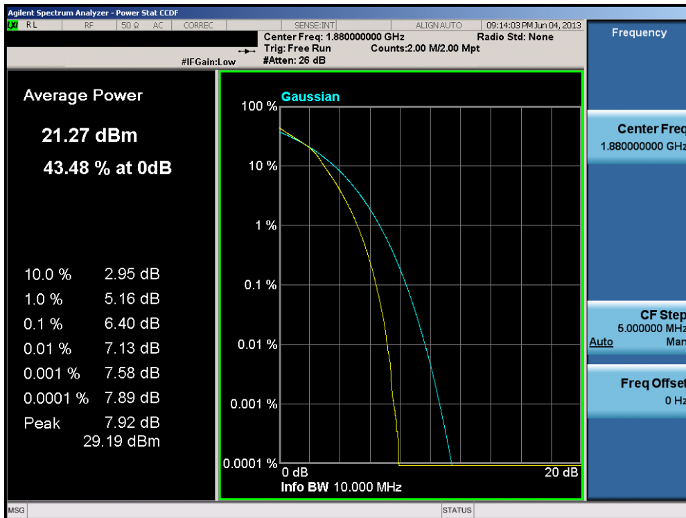
Plot 9-16. PAR Plot (10.0MHz 16-QAM – RB Size 50)
