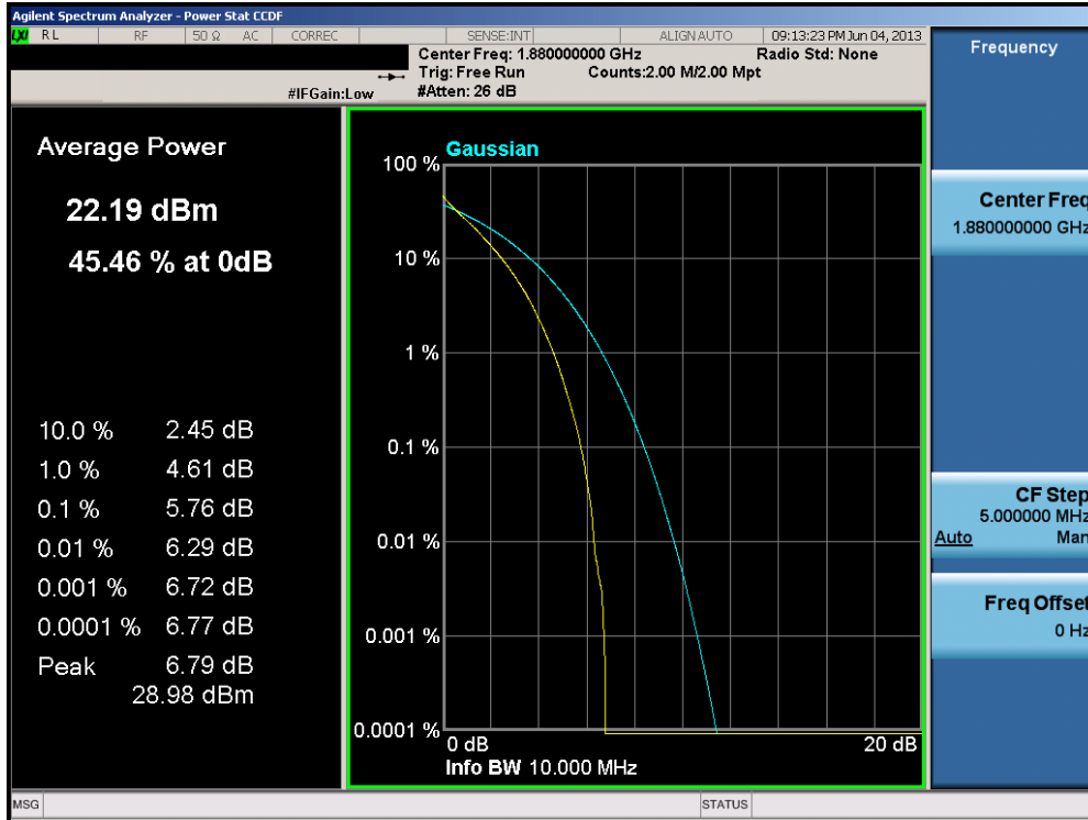
Plot 9-15. PAR Plot (10.0MHz QPSK – RB Size 50)
