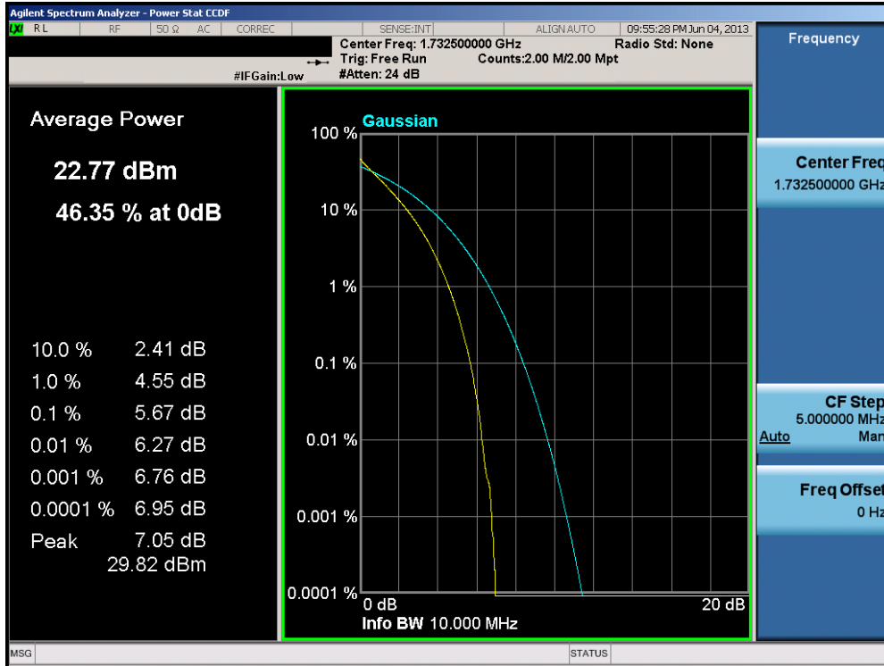
Plot 8-19. PAR Plot (10.0MHz QPSK – RB Size 50)
