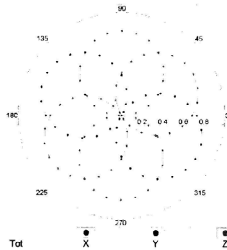
f=1800 MHz,R22
