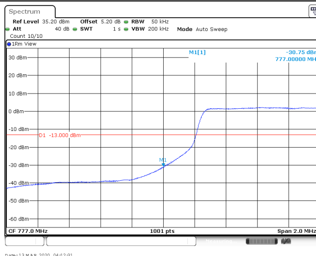
Band13 5MHz QPSK 23255 1RB#24
