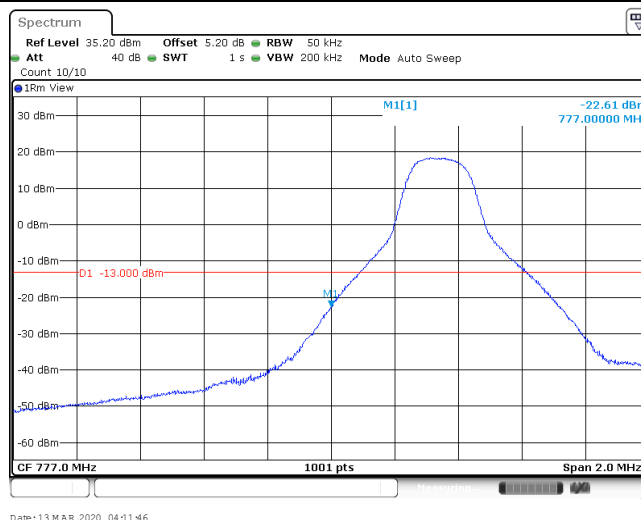
Band13 5MHz QPSK 23205 25RB#0
