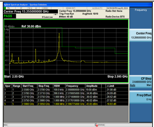
Band7-20MHz-QPSK-21350-1RB#99-PASS
