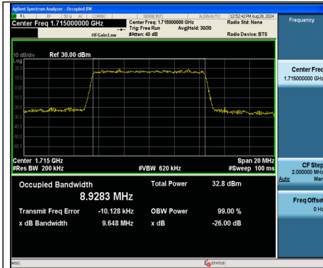
Band4-10MHz-QPSK-20000-50RB#0-PASS
