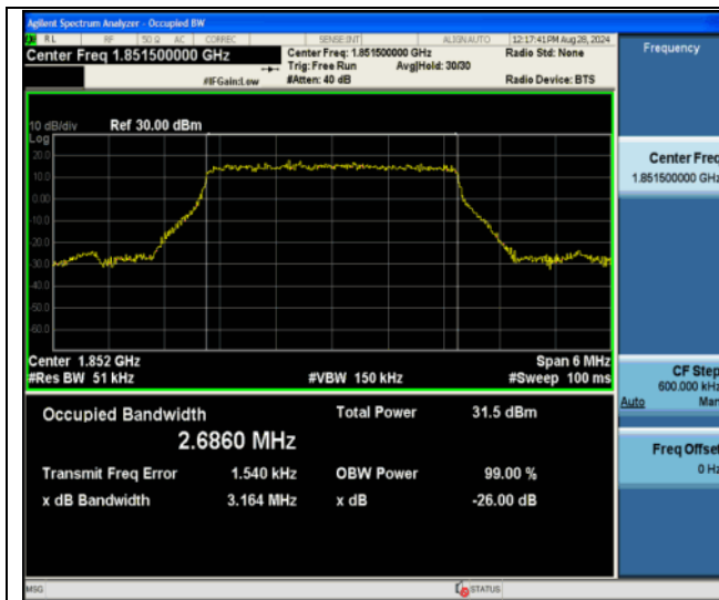
Band2-3MHz-QPSK-18615-15RB#0-PASS
