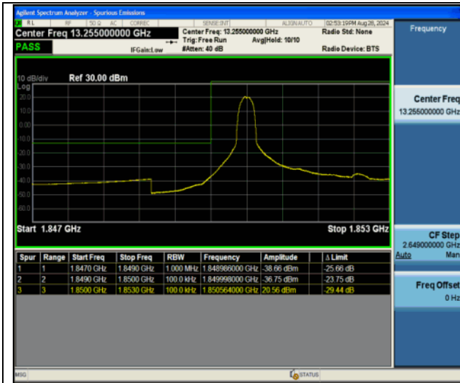
Band2-10MHz-QPSK-18650-1RB#0-PASS
