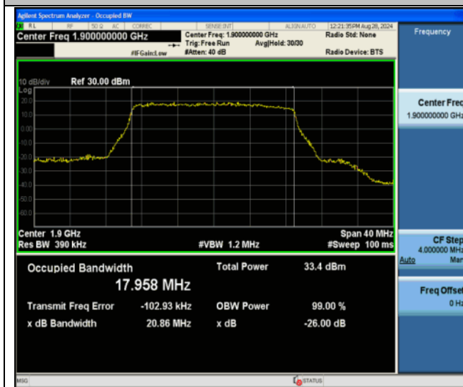
Band2-20MHz-QPSK-19100-100RB#0-PASS
