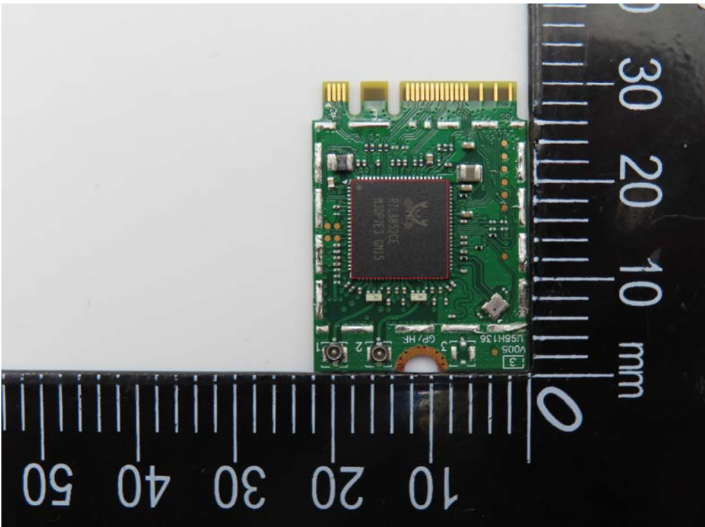
WLAN Module
