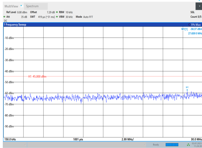
Band38-20MHz-QPSK-37850-1RB#0-Range2:0.15~30MHz
