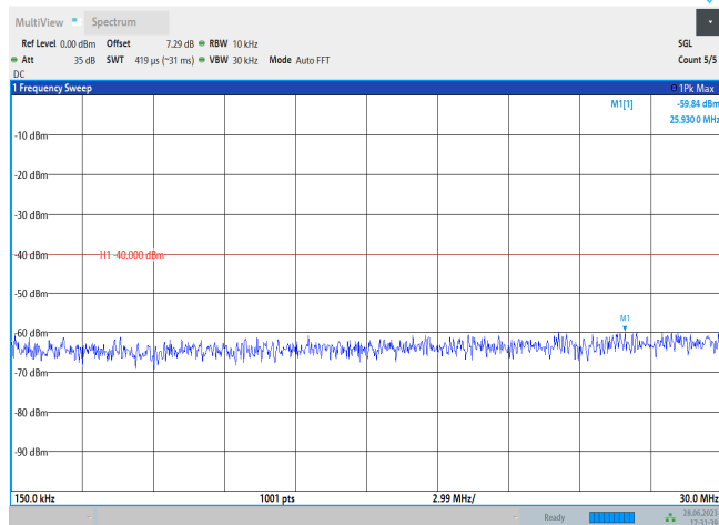
Band30-10MHz-QPSK-27710-1RB#0-Range2:0.15~30MHz
