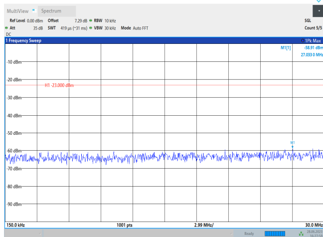
Band14-10MHz-QPSK-23330-1RB#0-Range2:0.15~30MHz
