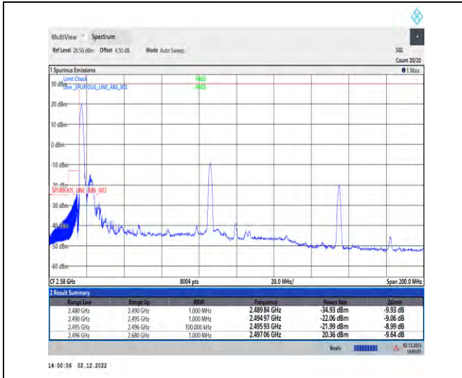
1-41-41-30-80+60-L-5-CP-QPSK-Edge_1RB_Left
