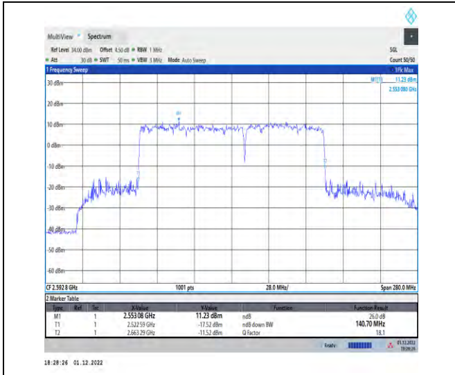
1-41-41-80+60-M-7-DFT-QPSK-Outer_Full
