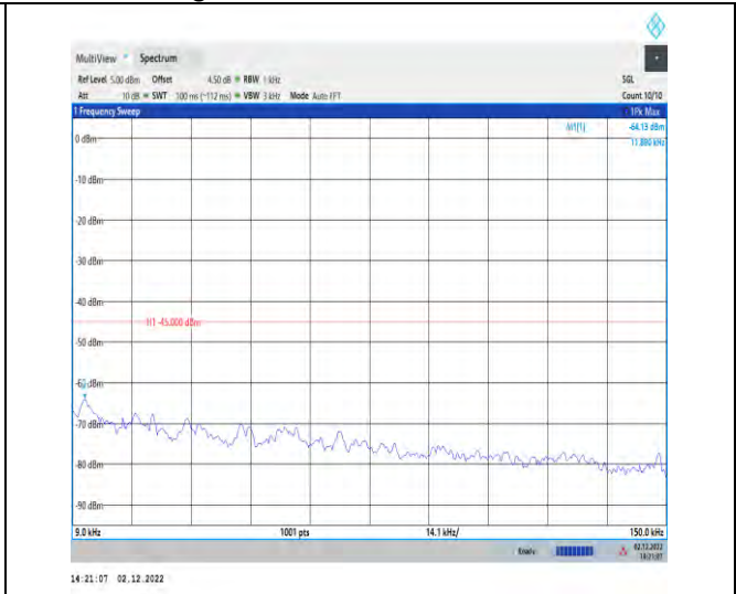
1-41-41-30-100-L-1-DFT-QPSK-Inner_1RB_Left-1@ 1-9-150
