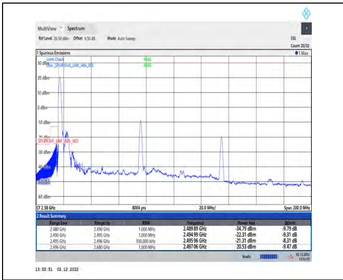
1-41-41-30-80+40-L-1-DFT-QPSK-Edge_1RB_Left
