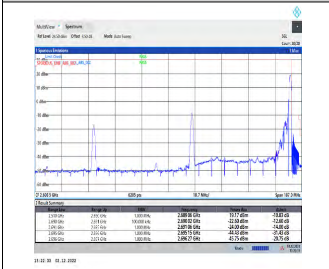
1-41-41-30-80+60-H-1-DFT-QPSK-Edge_1RB_Right
