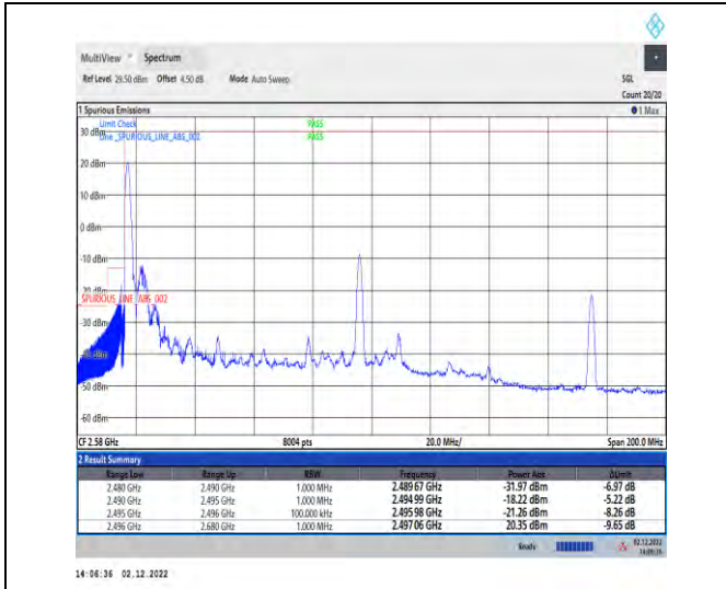
1-41-41-30-100+60-L-5-CP-QPSK-Edge_1RB_Left
