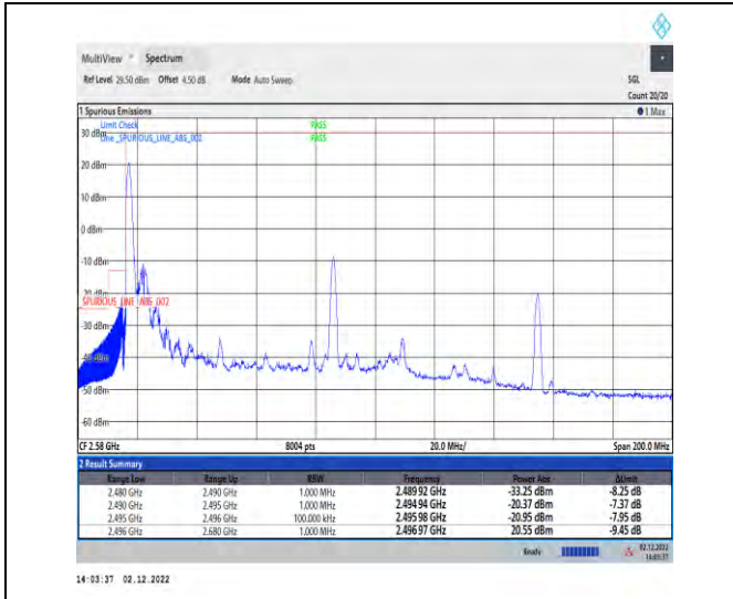
1-41-41-30-100+40-L-5-CP-QPSK-Edge_1RB_Left
