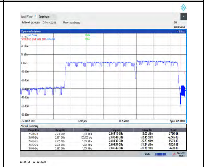
1-41-41-30-80+50-H-3-DFT-QPSK-Outer_Full
