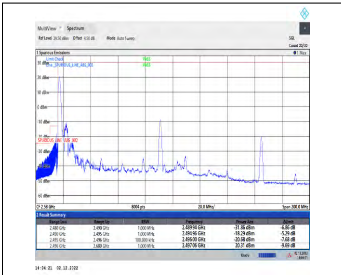
1-41-41-30-100+50-L-4-CP-QPSK-Edge_1RB_Left
