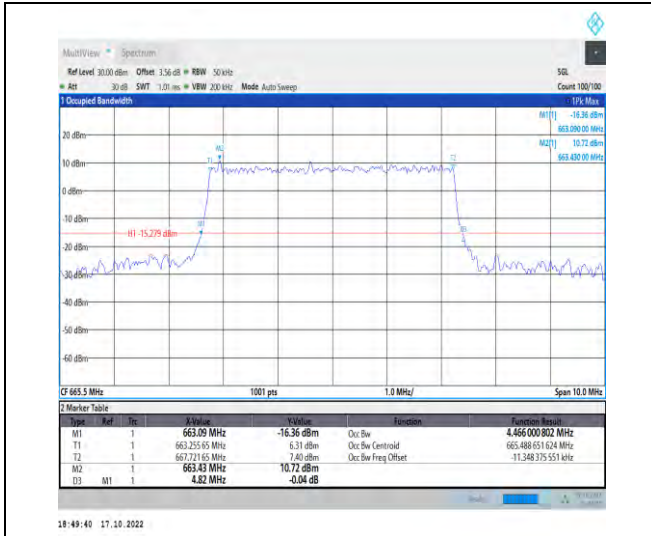
1-N71-PC3-15-5-L-6-CP-QPSK-Outer_Full-25@0-A Ant1-4.466-4.820-≤5-PASS
