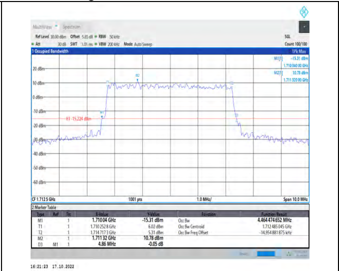
1-N66-PC3-15-5-L-7-CP-16QAM-Outer_Full-25@0-A Ant1-4.464-4.860-≤5-PASS
