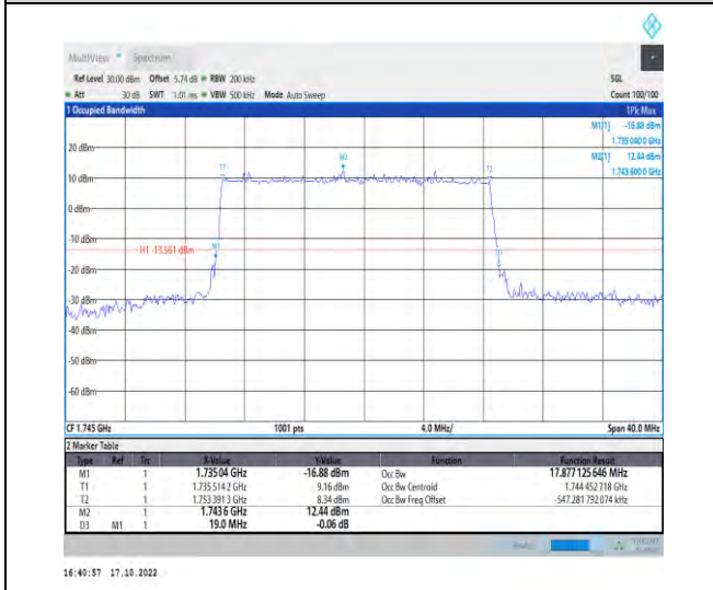
1-N66-PC3-15-20-M-4-DFT-64QAM-Outer_Full-100@0-Ant1-17.877-19.000-≤20-PASS
