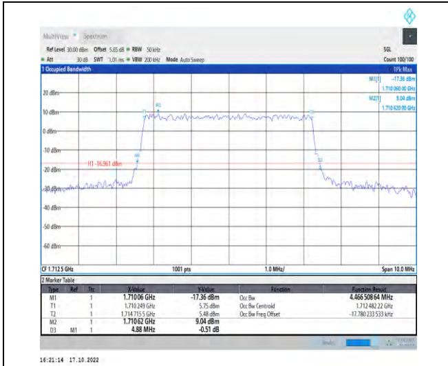
1-N66-PC3-15-5-L-6-CP-QPSK-Outer_Full-25@0-A Ant1-4.467-4.880-≤5-PASS
