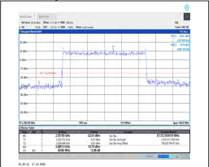
1-N41-PC2-30-70-M-7-CP-16QAM-Outer_Full-189@ 0-Ant1-67.513-69.860-≤70-PASS
