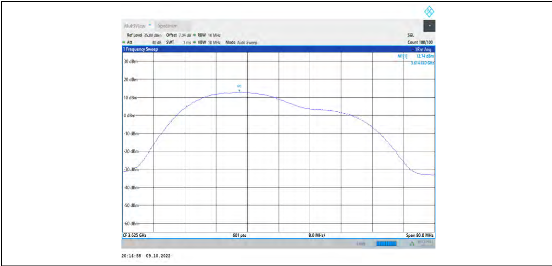
48-48-20MHz-20MHz-QPSK-QPSK-55891-56089-1RB#0-ORB#0
