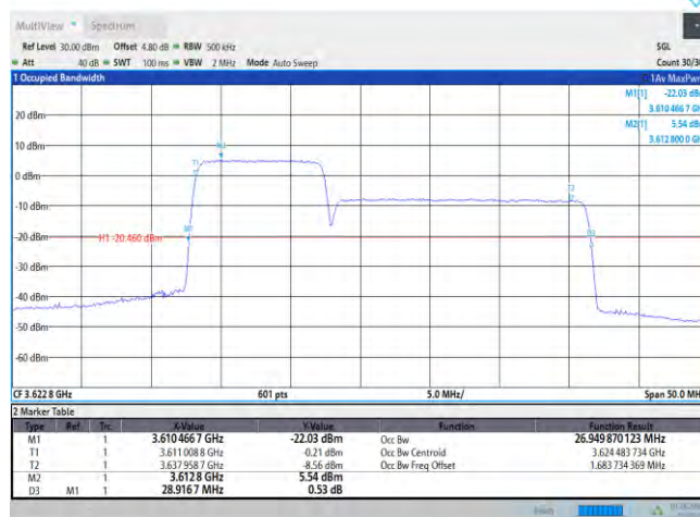
48-48-10MHz-20MHz-QPSK-QPSK-55896-56040-50RB#0-100RB#0
