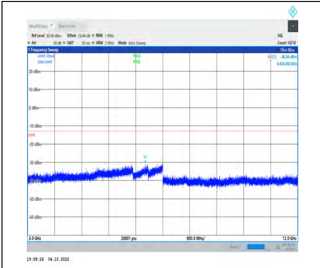
1-N25-PC3-15-40-L-1-DFT-QPSK-Inner_1RB_Left-1 @1-3000-12000-Ant1-6924.45--30.56--13-PASS
