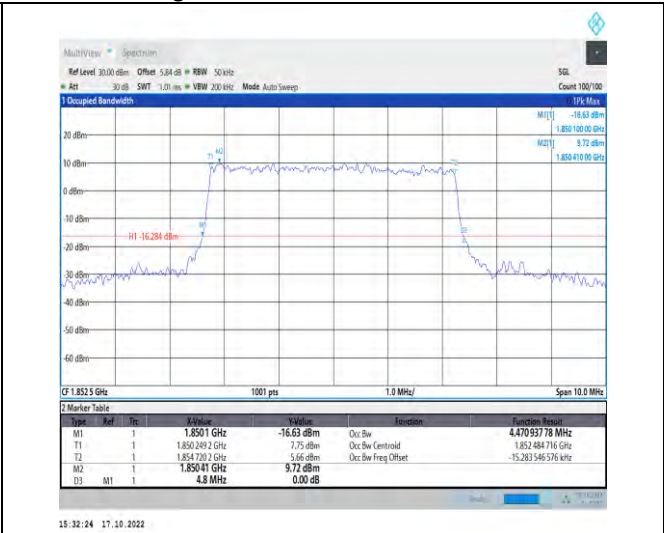
1-N25-PC3-15-5-L-7-CP-16QAM-Outer_Full-25@0-A Ant1-4.471-4.800-≤5-PASS
