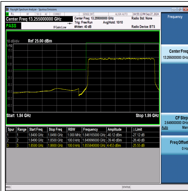
NTNV_N25_PC3_15_10_L_TID1_#1
