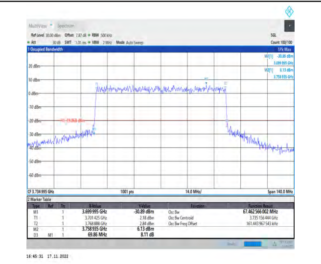
1-N78-3700-3800-PC2-30-70-L-7-CP-16QAM-Outer_Full-189@0-Ant1-67.463-69.860-≤70-PASS
