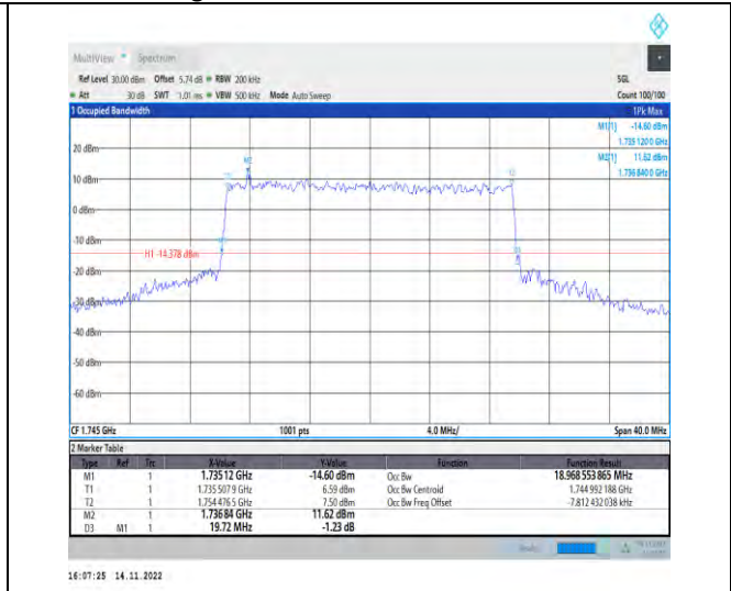
1-N66-PC3-15-20-M-8-CP-64QAM-Outer_Full-106@ 0-Ant1-18.969-19.720-≤20-PASS
