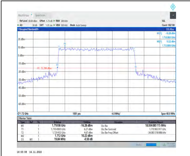
1-N66-PC3-15-20-L-8-CP-64QAM-Outer_Full-106@ 0-Ant1-18.934-19.840-<20-PASS
