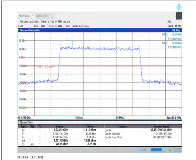
1-N66-PC3-15-40-M-1-DFT-QPSK-Outer_Full-216@ 0-Ant1-38.483-40.320-≤40-PASS
