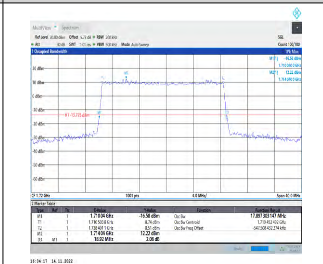
1-N66-PC3-15-20-L-3-DFT-16QAM-Outer_Full-100 @0-Ant1-17.897-18.920-≤20-PASS
