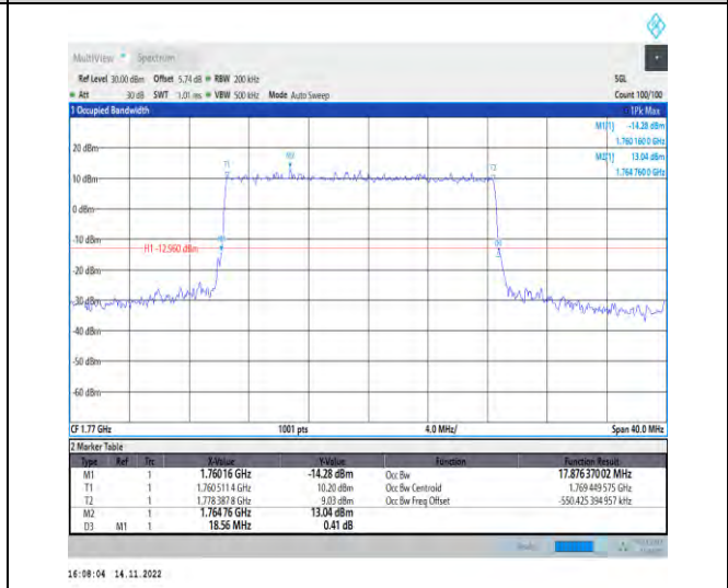
1-N66-PC3-15-20-M-1-DFT-QPSK-Outer_Full-100@ 0-Ant1-17.876-18.560-≤20-PASS
