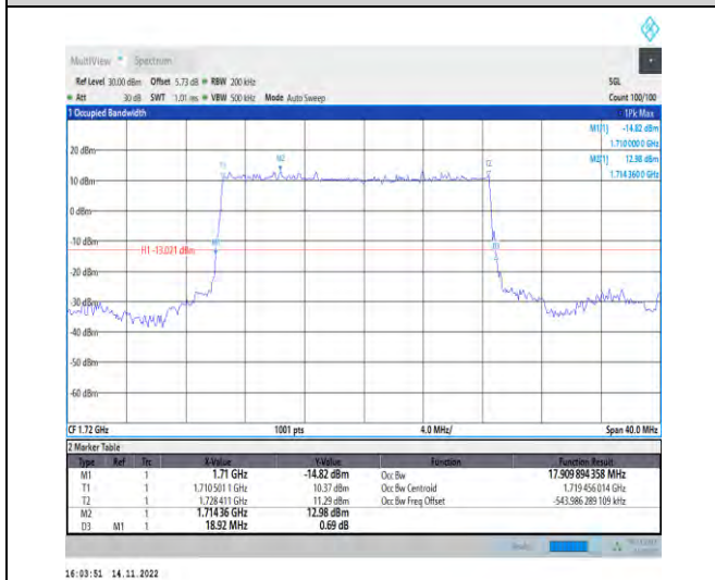
1-N66-PC3-15-20-L-2-DFT-PI2BPSK-Outer_Full-100 @0-Ant1-17.91-18.920-≤20-PASS
